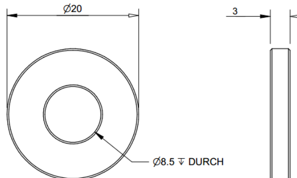
Abb. 1: Dimensionen der Platzhalter-Unterlagescheibe (ADEC Part. # 70109)
