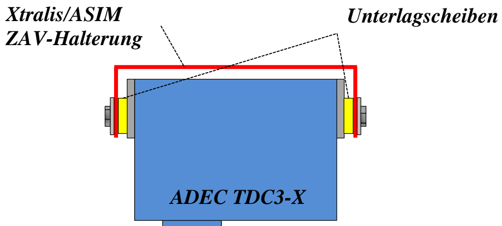
Abb. 2: Front-Ansicht eines TDC3 in einer ZA V 290-L1 Halterung
