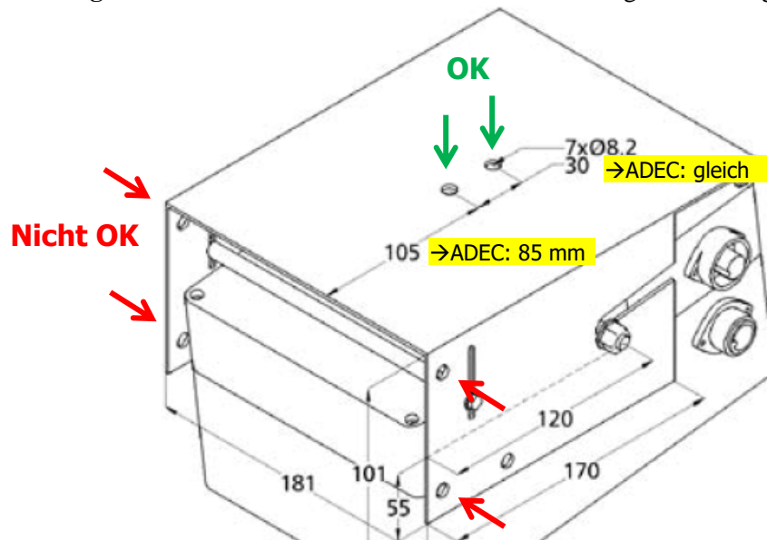
Abb. 3: Xtralis/ASIM ZA V 290-L1 Halterung (©Xtralis) Original Dokument siehe https://xtralis.com/file.cfm?id=496
