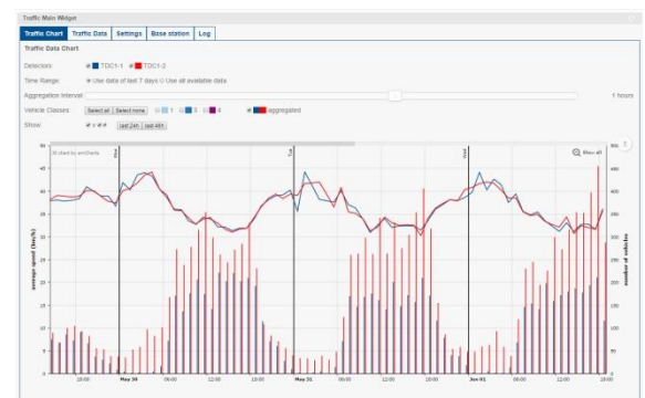
Internetbrowser-Ansicht von stündlichen Mittelwerten des Verkehrsvolumens und der Geschwindigkeit
